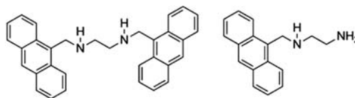
図 1 芳香族化合物の構造 (左) diAntED (右) monoAntED
