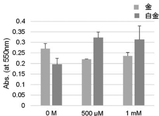
図2 diAntED の反応溶液における UV-vis 吸収スペクトル
