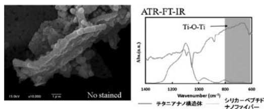
Figure 4 チタニアナノ構造体の FE-SEM 像と ATR-FT-IR.
