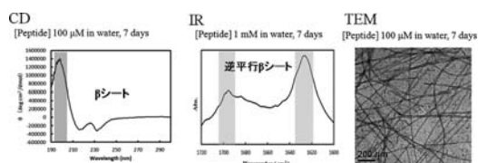
Figure 2 RU019 の CD, ATR-FT-IR, TEM 像。
