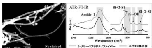
Figure 3 シリカーペプチド複合体の FE-SEM 像と ATR-FT-IR.
