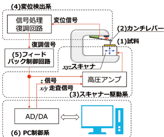
原子間力顕微鏡の基本装置構成
