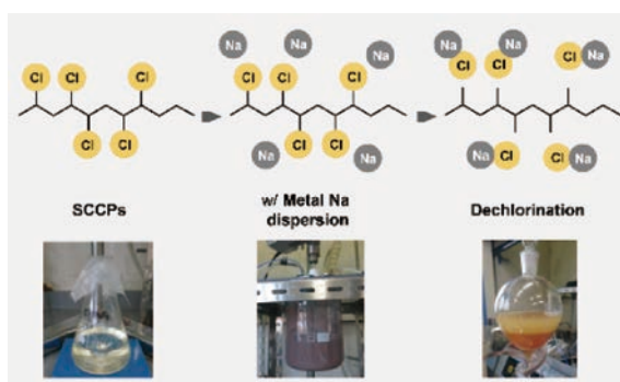
SCCPs の化学処理
